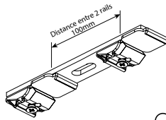
Support plafond double blanc long (espace 100mm)
